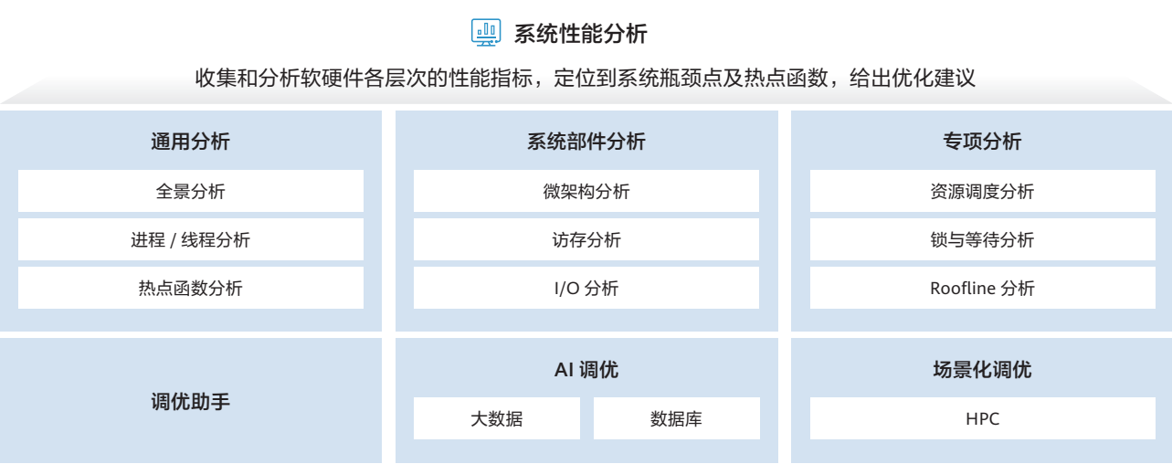
图 3-43 系统性能分析工具
