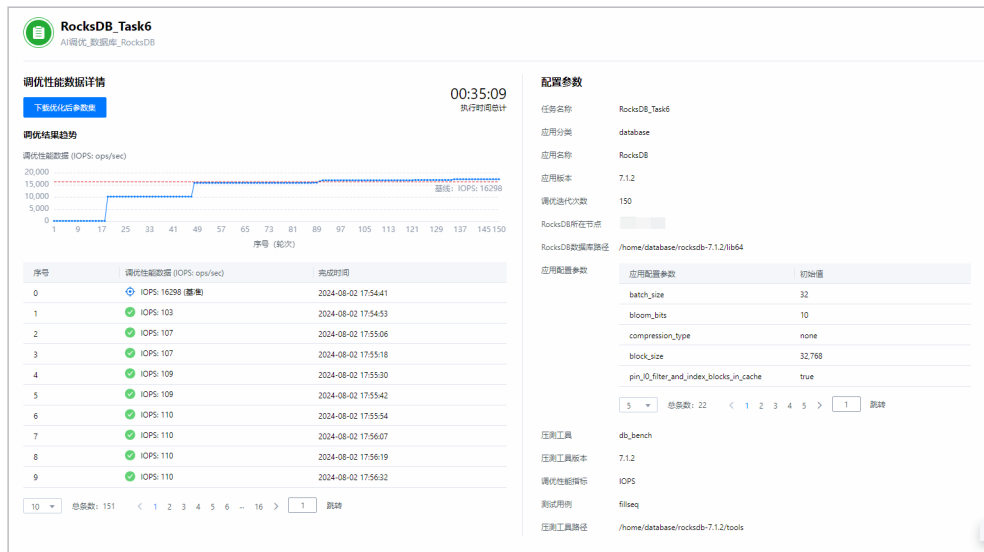
图 3-62 下载优化后参数集
