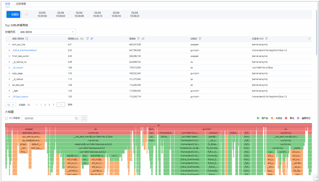
图 3-47 热点函数分析结果
