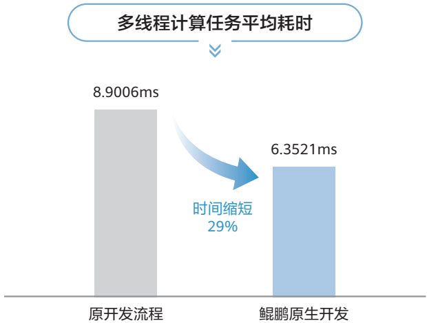
图 4-18 高效计算引擎多线程计算任务平均耗时对比
