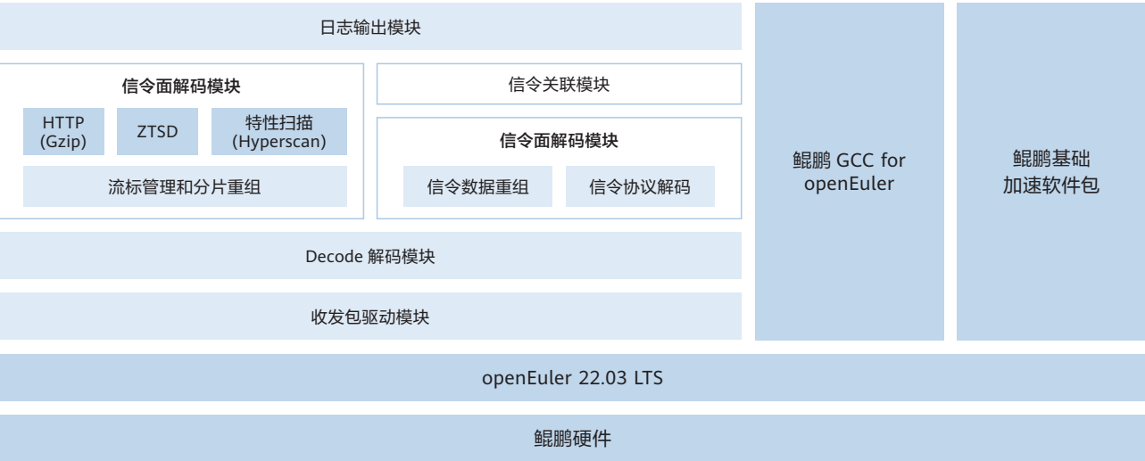
图 4-9 恒安嘉新安全采集分析平台方案
