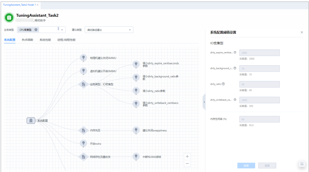
图 3-57 系统配置分析结果
