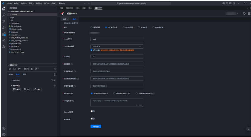
图 3-35 HPC 并行应用参数配置
