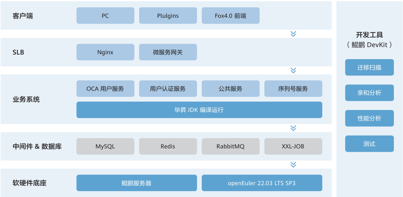
图 4-3 分布式企业网银系统 & 远程经营服务平台 鲲鹏原生架构图
