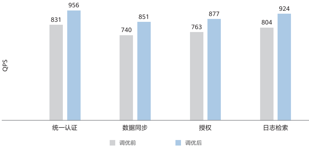
图 4-22 调优前后典型场景性能对比测试
