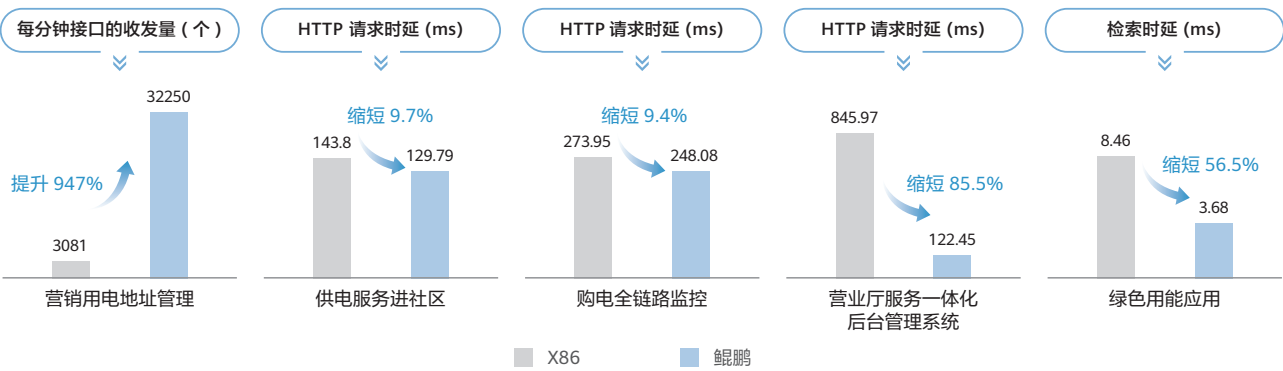
图 4-16 5 款软件原生开发改造后性能对比
