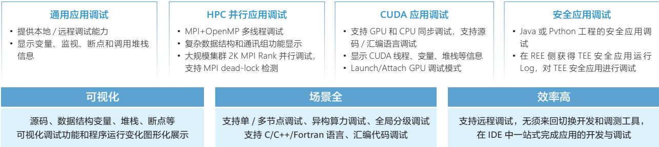
图 3-32 编译调试工具
