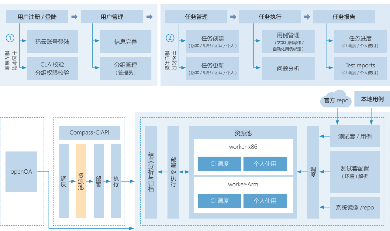
图 3-92 EulerTest 测试管理平台
