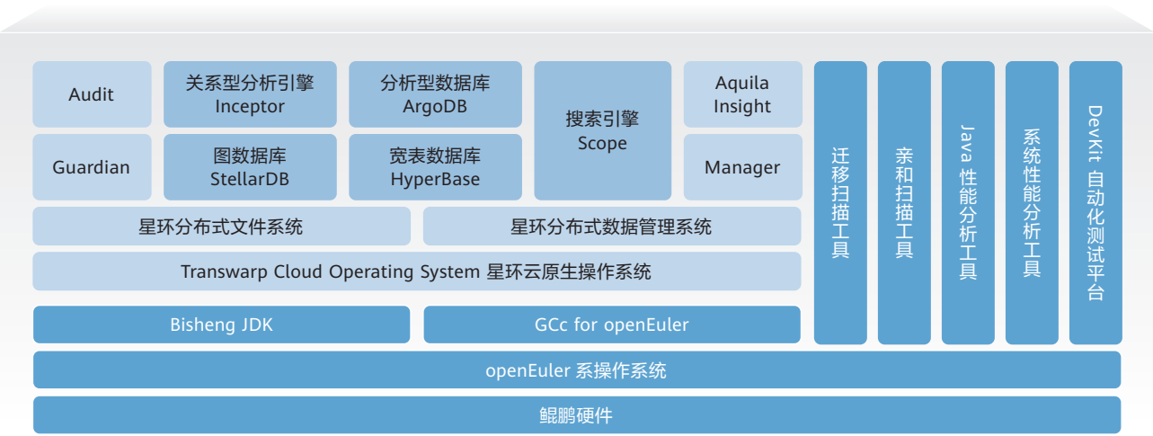
图 4-23 星环大数据基础平台 TDH 原生开发架构图
