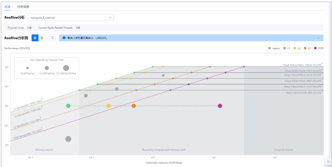
图 3-55 Roofline 分析结果
