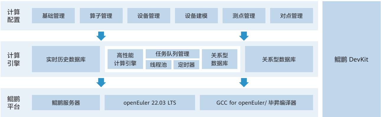
图 4-17 新能源计算平台基于鲲鹏的原生开发框架
