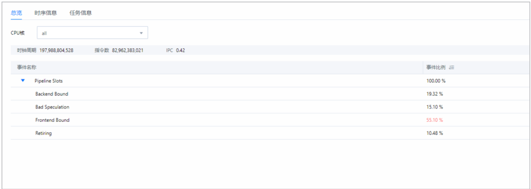
图 3-49 微架构分析结果
