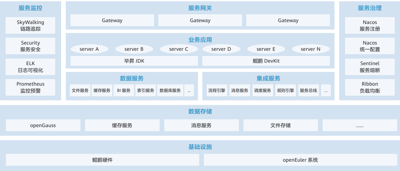
图 4-21 东华软件基于鲲鹏原生应用开发框架
