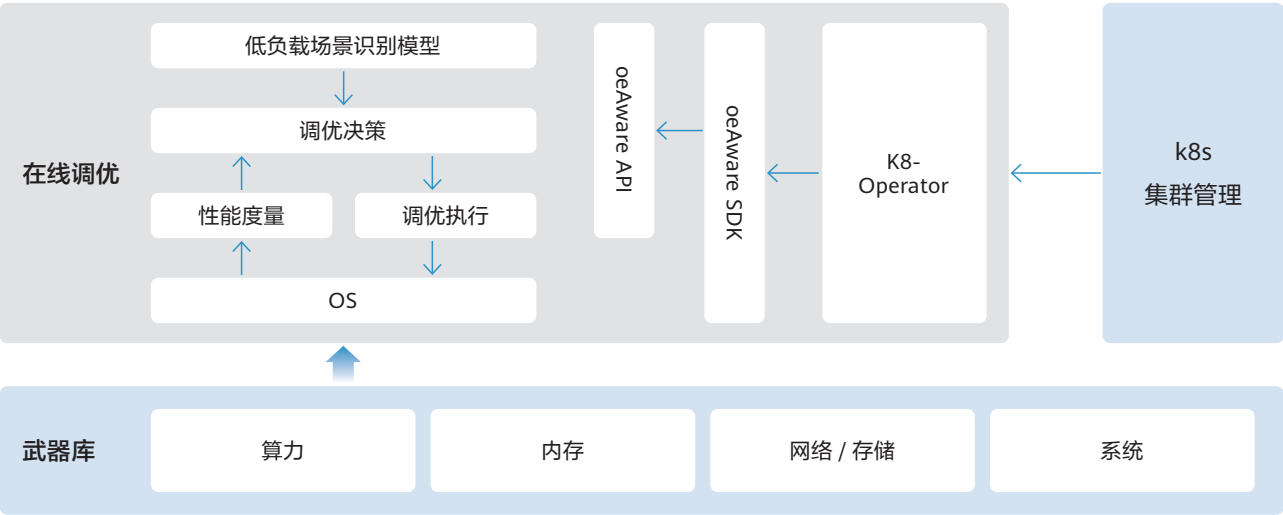
图 3-90 oeAware 调优框架
