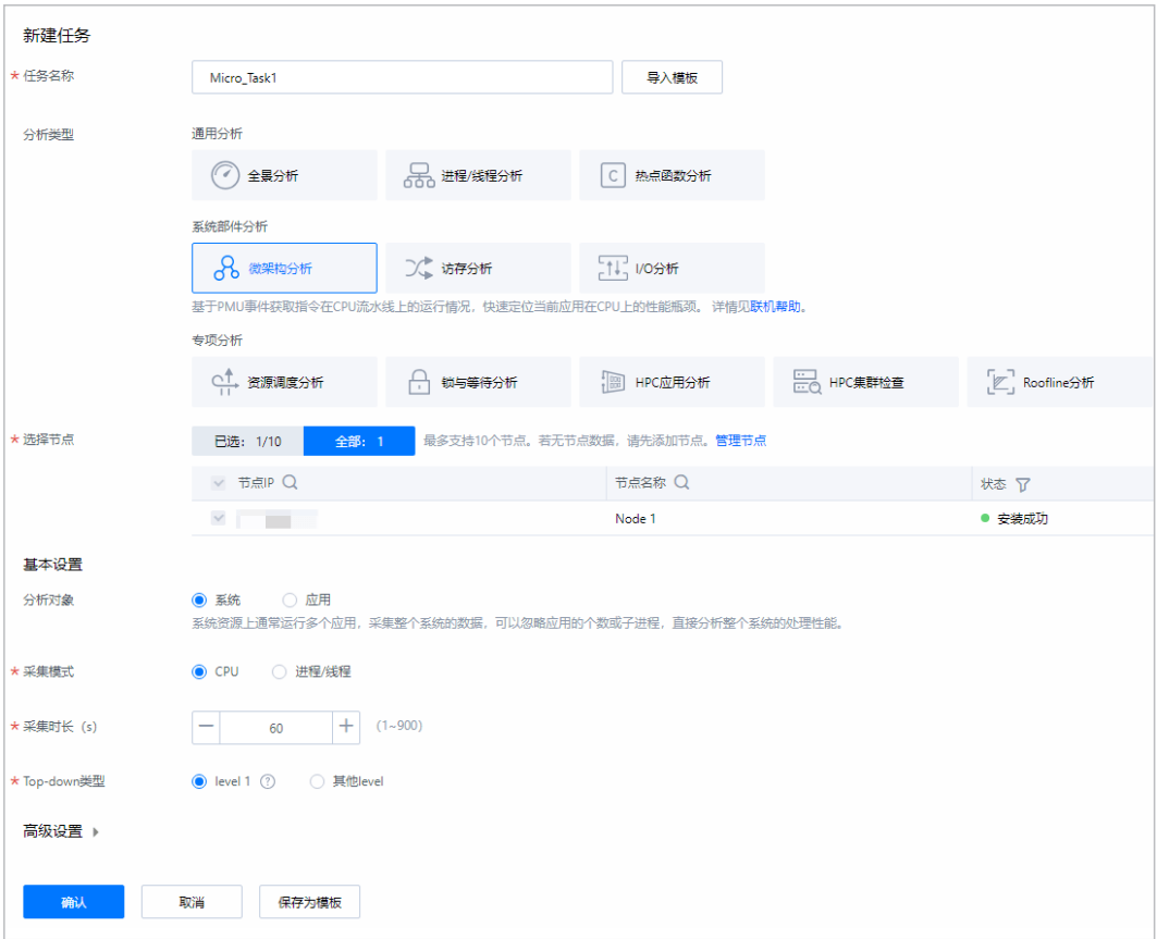
图 3-48 系统部件分析
