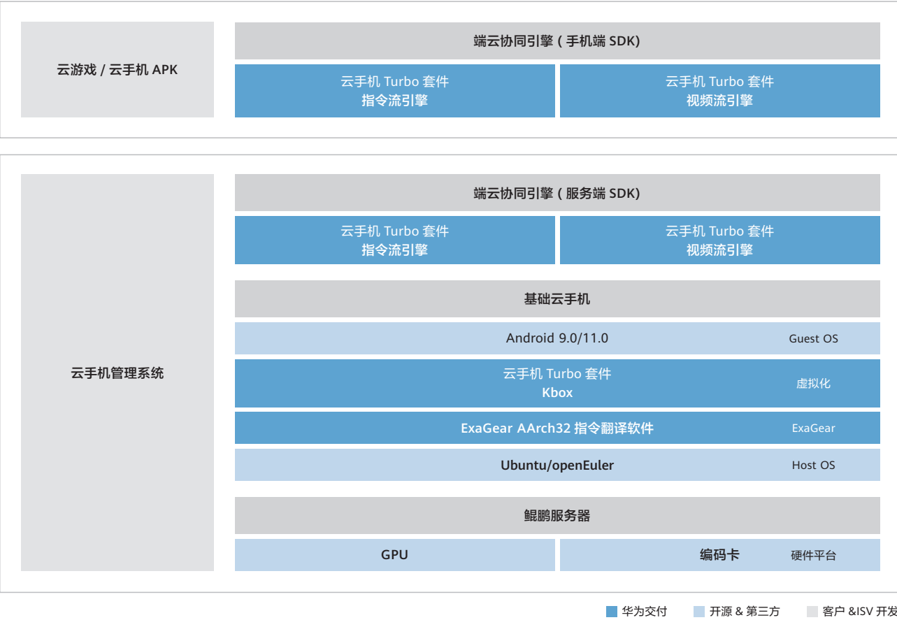
图 3-16 鲲鹏 BoostKit ARM 原生云手机整体架构
