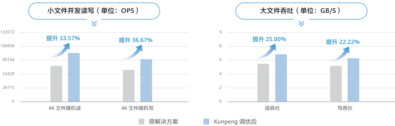
图 4-27 鲲鹏优化前后性能对比
