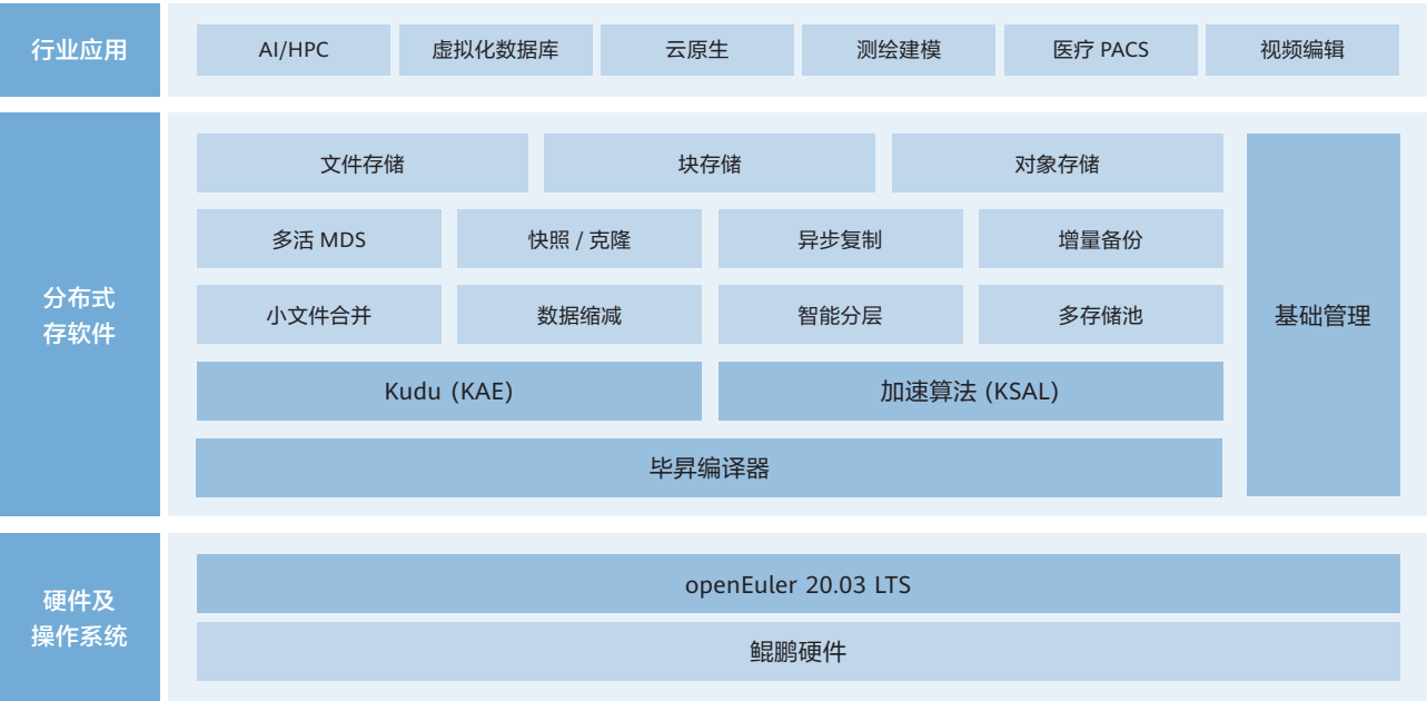
图 4-25 分布式存储 EDS 的鲲鹏原生架构图
