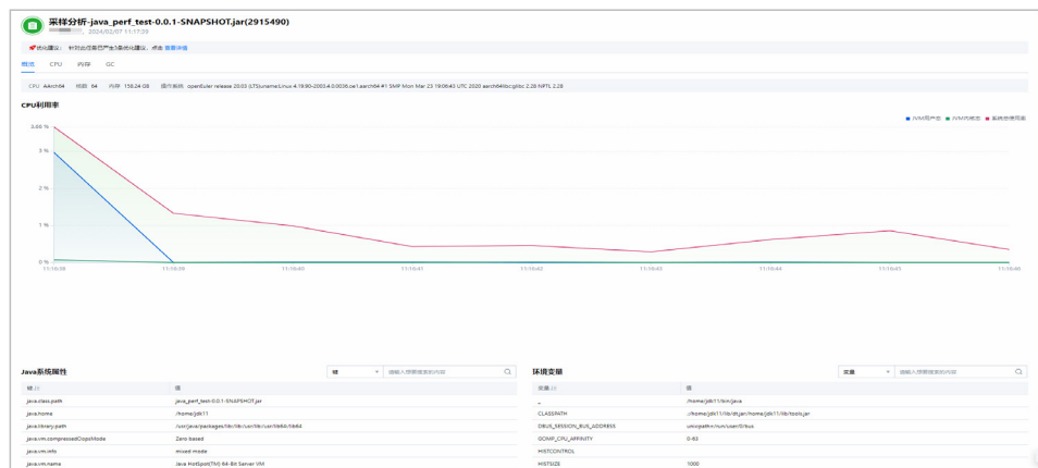
图 3-70 查看采样分析结果
