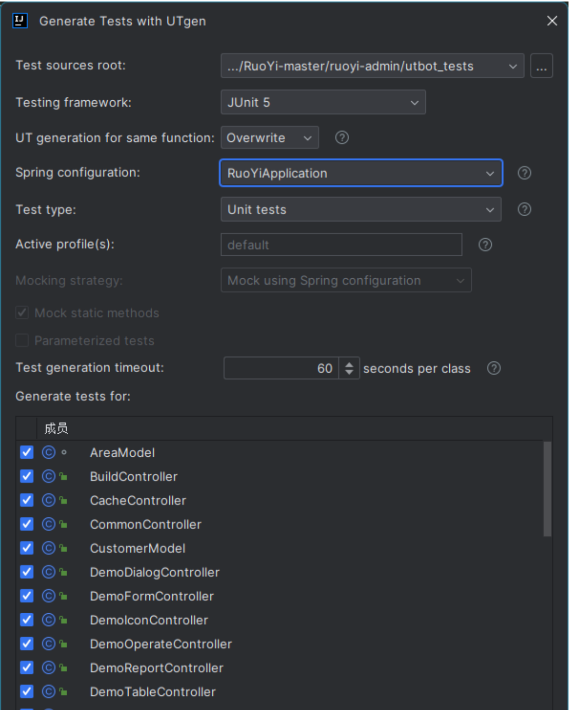
图 3-21 基于 SpringBoot 项目
