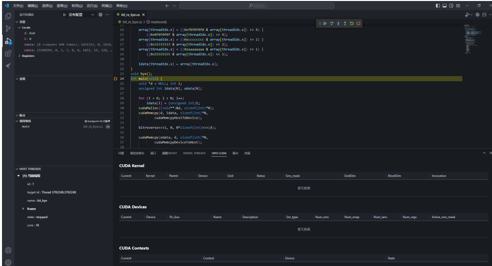
图 3-39 CUDA 应用调试
