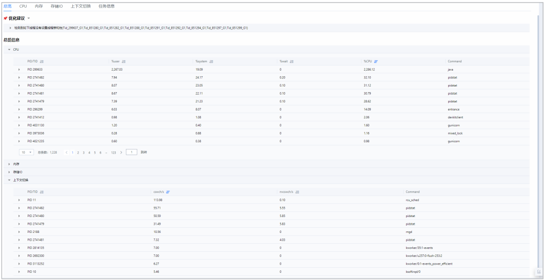
图 3-46 进程 / 线程分析结果
