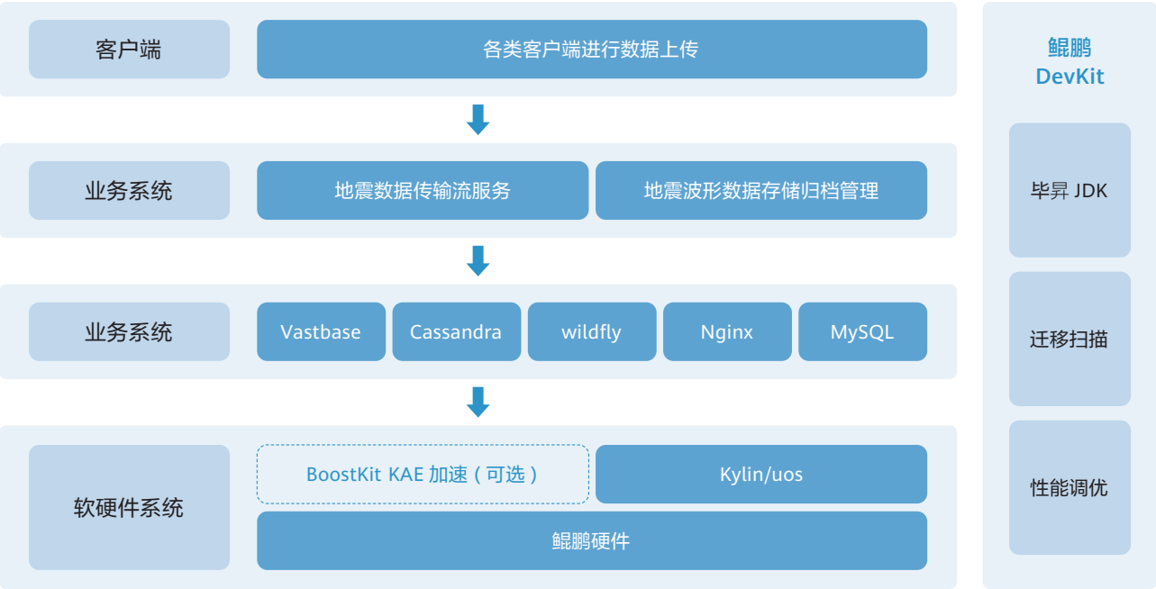
图 4-13 SeisWave-SSS 和 SeisWave-AWS 鲲鹏原生架构图
