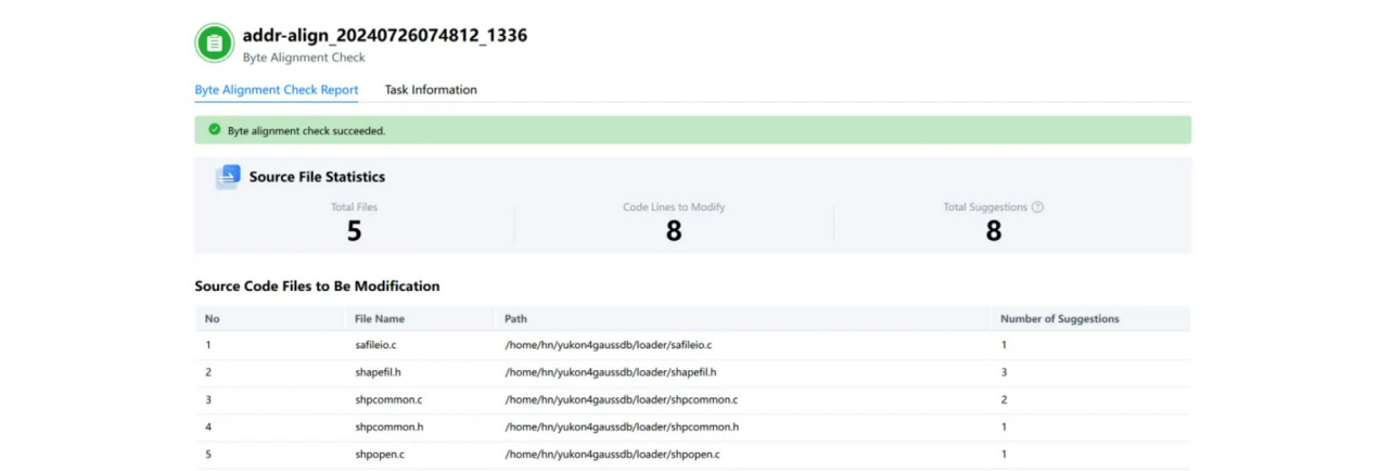
图 4-11 迁移扫描门禁检查报告
